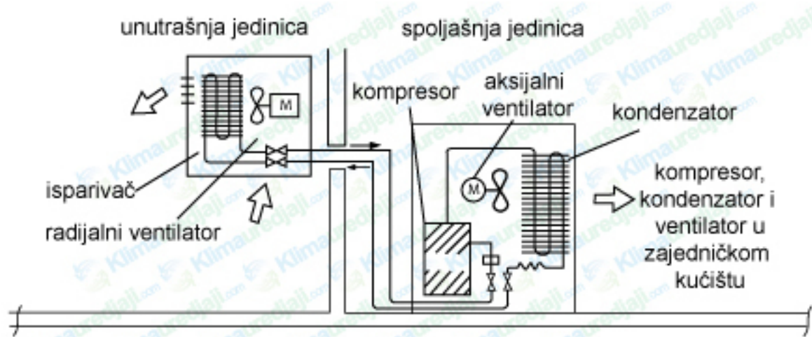
Blok šema
